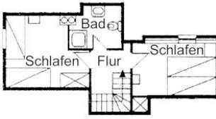
Grundriss Obergeschoß
